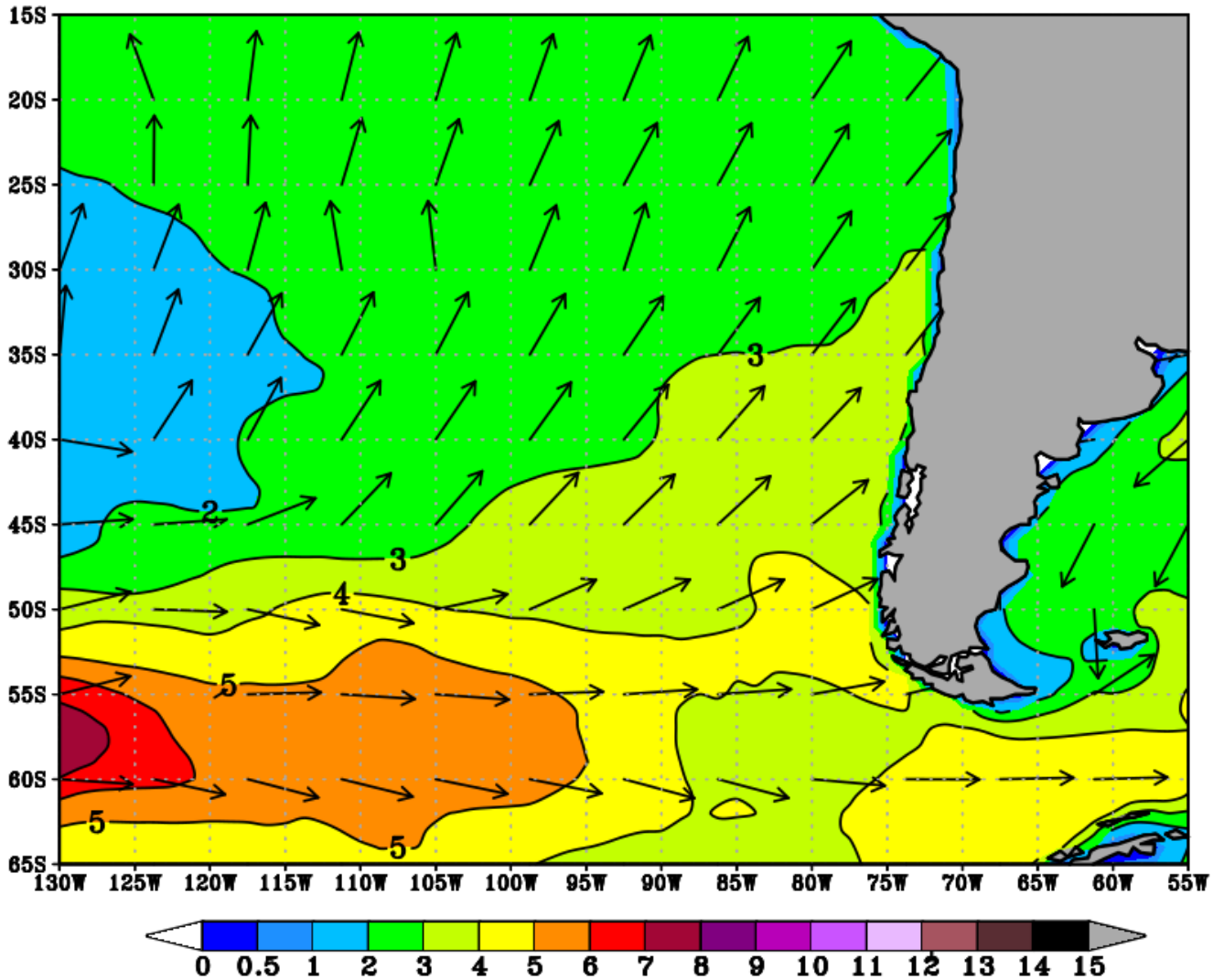
ALTURA DE OLA SIGNIFICATIVA, EN METROS Datos grib Modelo Global NWW3 corrida 06Z12FEB2021 res 0.5°x0.5° procesado con GrADS
